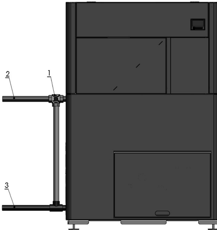
1. Mešni ventil 2. Polazni vod 3. Povratni vod
