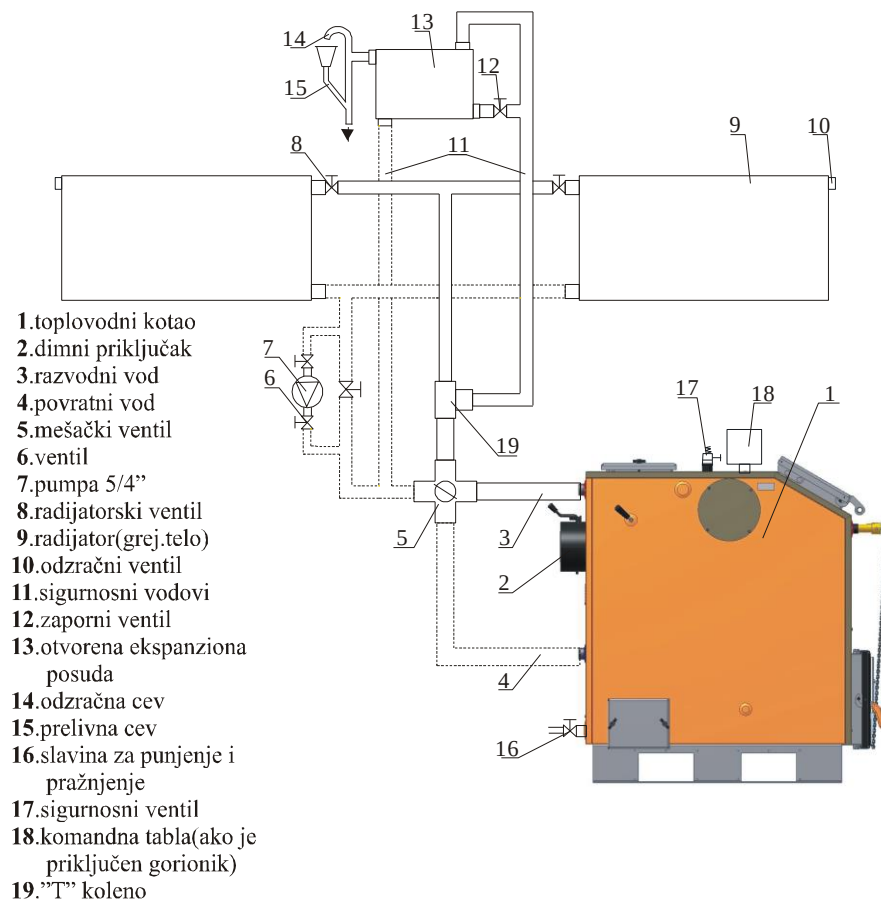
-otvoreni sistem grejanja – šema
