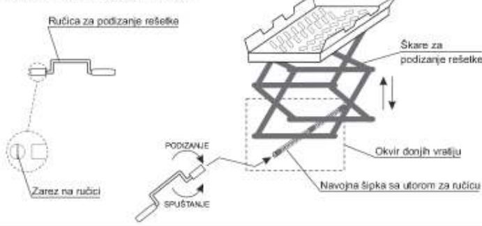
Slika 6. - Rad sa rešetkom u ložištu
