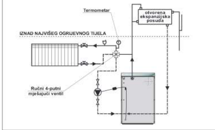
Shema 1. - Prikaz spajanja kotla na otvoreni sustav grijanja BIO-CET 23, 29 B
