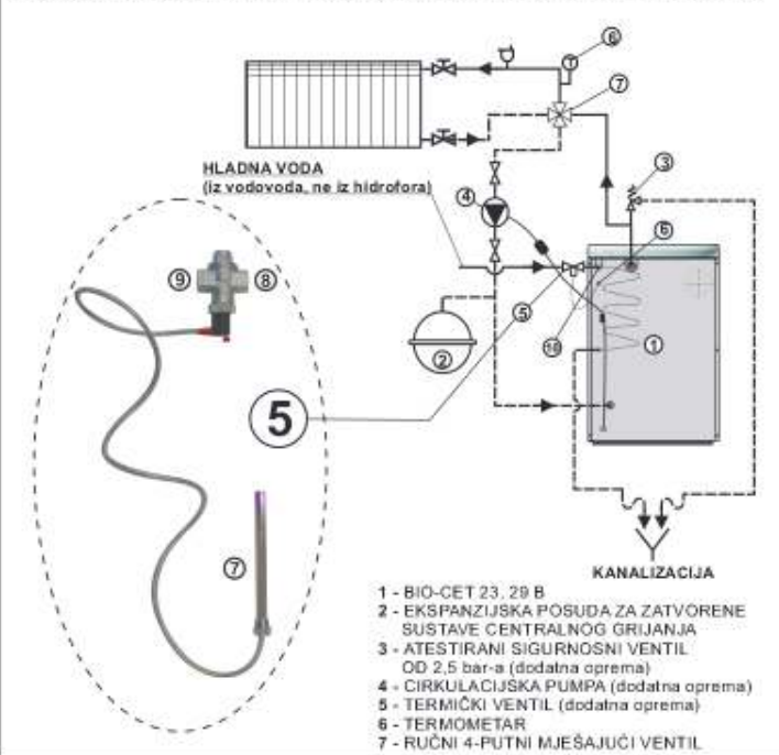
Shema 2. - Prikaz spajanja kotla na zatvoreni sustav grijanja BIO-CET 23, 29 B - lijeva izvedba
