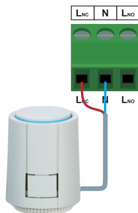
NC Actuator
