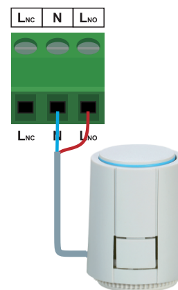
NO Actuator
